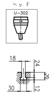
A部 T溝詳細図 SCL 1:5
