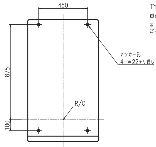
B-B図：アンカー穴寸法図
