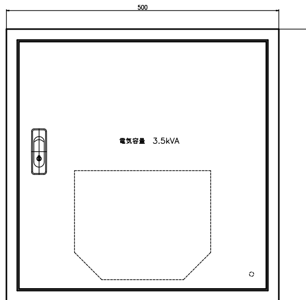
制御盤
