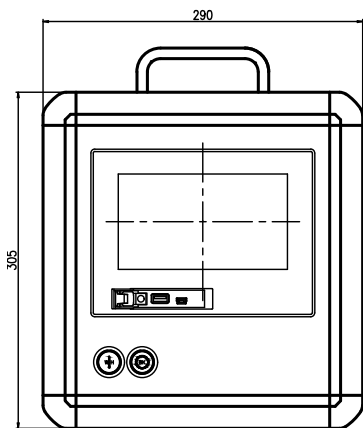
操作盤
